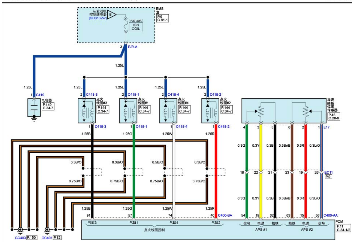
发动机控制系统(G4FJ: GAMMA 1.6L T-GDI A/T)(6)
